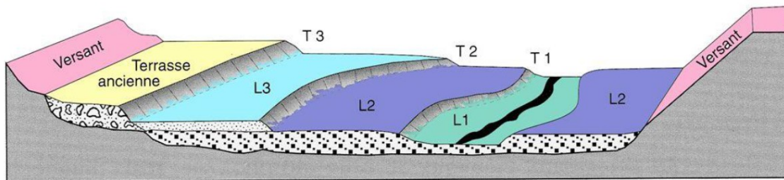
Figure 55 : Schéma d'une plaine alluviale type © Masson Garry Ballais modifié par SIEE
